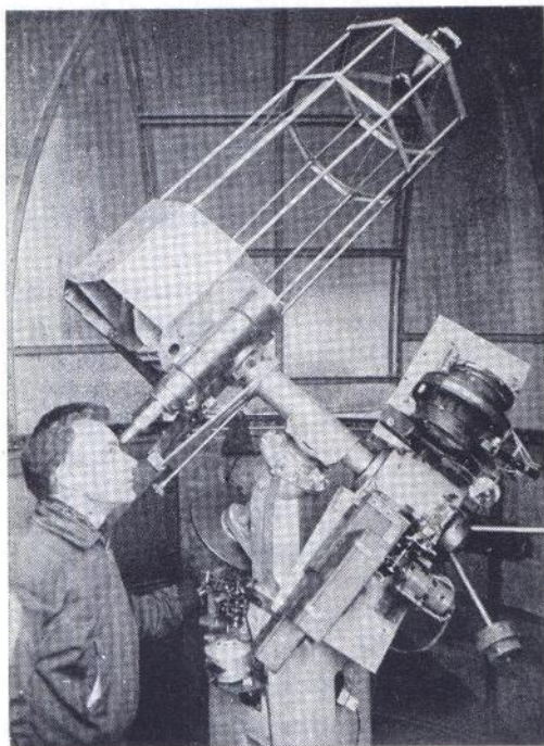
Installation astronomique réalisée par P. Bourge. Télescope équatorial Cassegrain de 400 mm. En bas, à droite, se trouve un dispositif destiné à filmer les éclipses.
